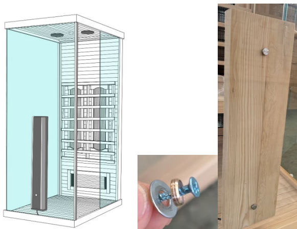
(7) Asambleati cutia de încălzire din față, Folosești șuruburi 4x20
